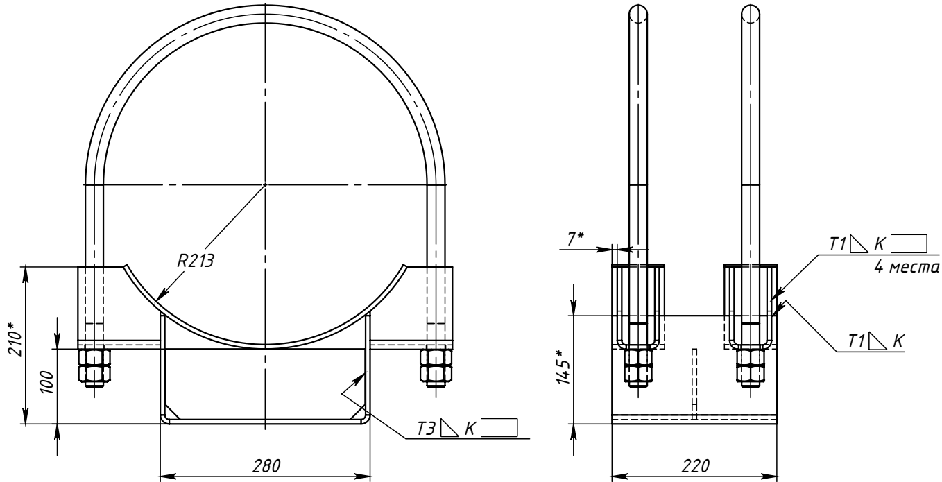
Поз.2 (Ложемент)
