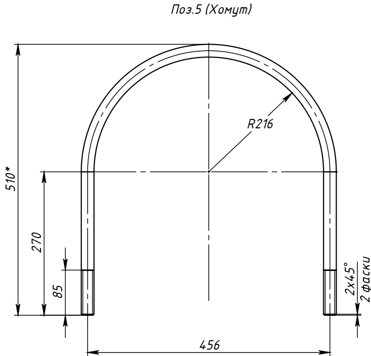
Поз.5 (Хомут)
